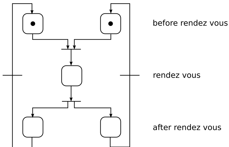
Figure 2-32. Rendez Vous Petri Net
